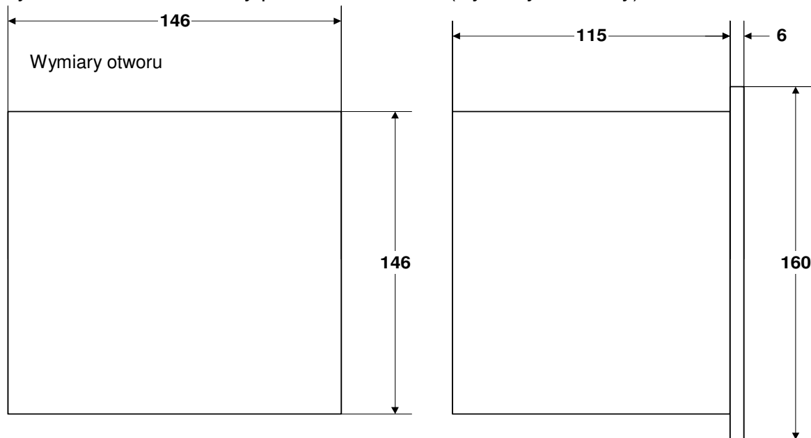
Rys. 5. Otwór montażowy pod WP-EC 01-2a (wymiary obudowy)
