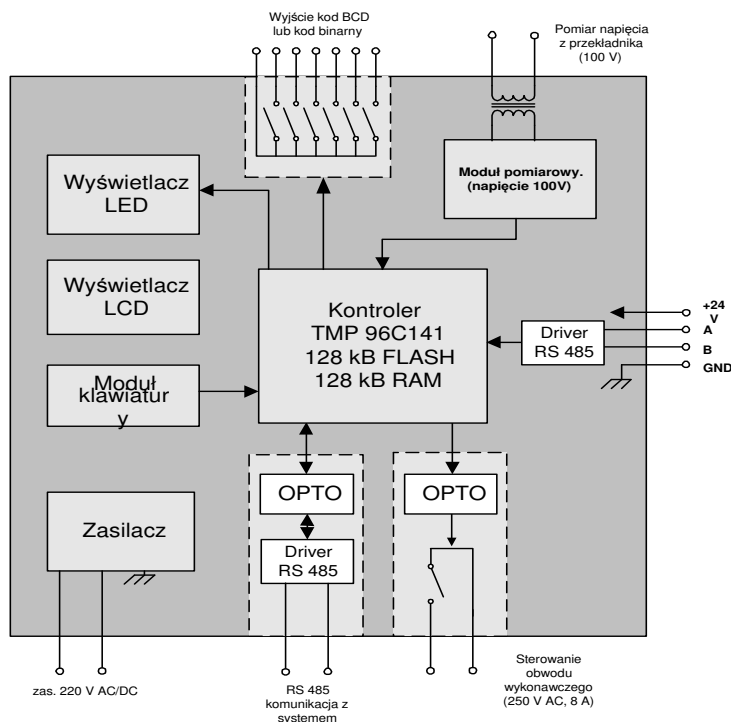
Rys. 2. Schemat blokowy odbiornika
