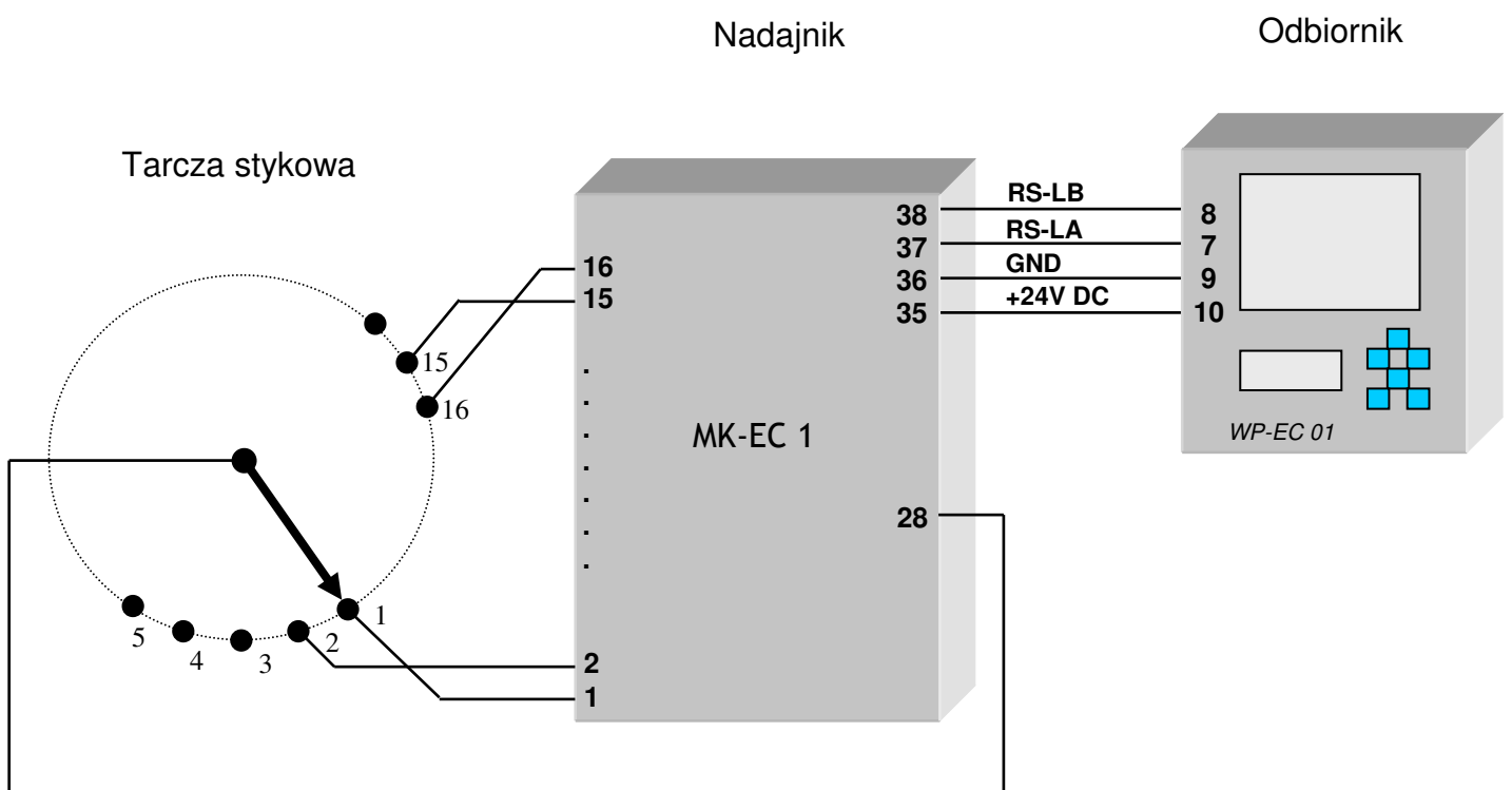
Rys. 4. Schemat podłączenia nadajnika do tarczy stykowej oraz do odbiornika WP-EC 01-2a
