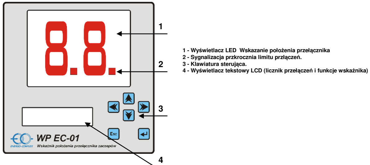
Rys. 7. Płyta czołowa WP-EC 01-2a
