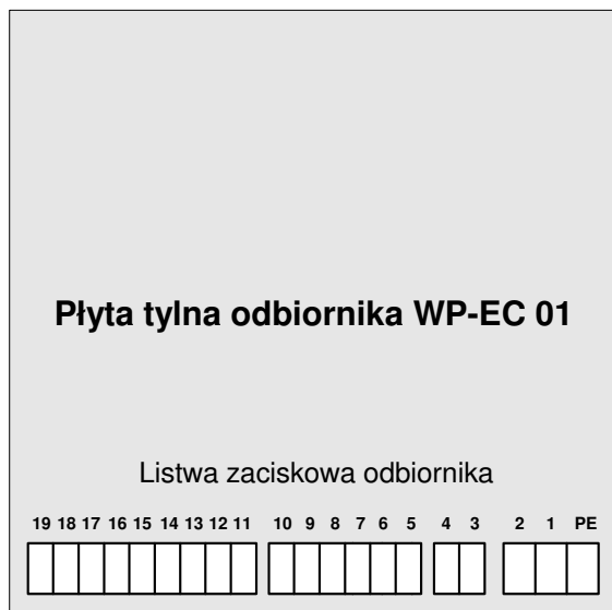
Rys. 6. Listwa połączeniowa WP-EC 01-2a
